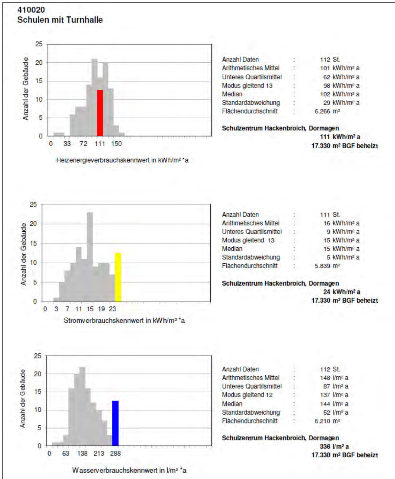
Abbildung 15: Verbrauchskennwerte nach ages [ages 2005]
