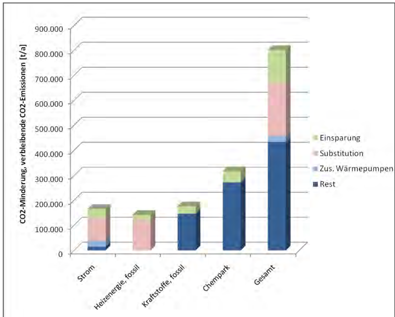
Abbildung 25: CO 2 -Minderungspotentiale nach Endenergieträgern [eigene Darstellung]
